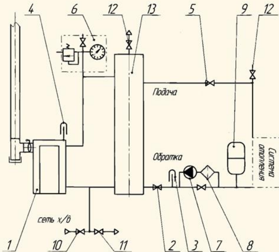
Схема подключения котла к закрытой системе с принудительной циркуляцией теплоносителя
