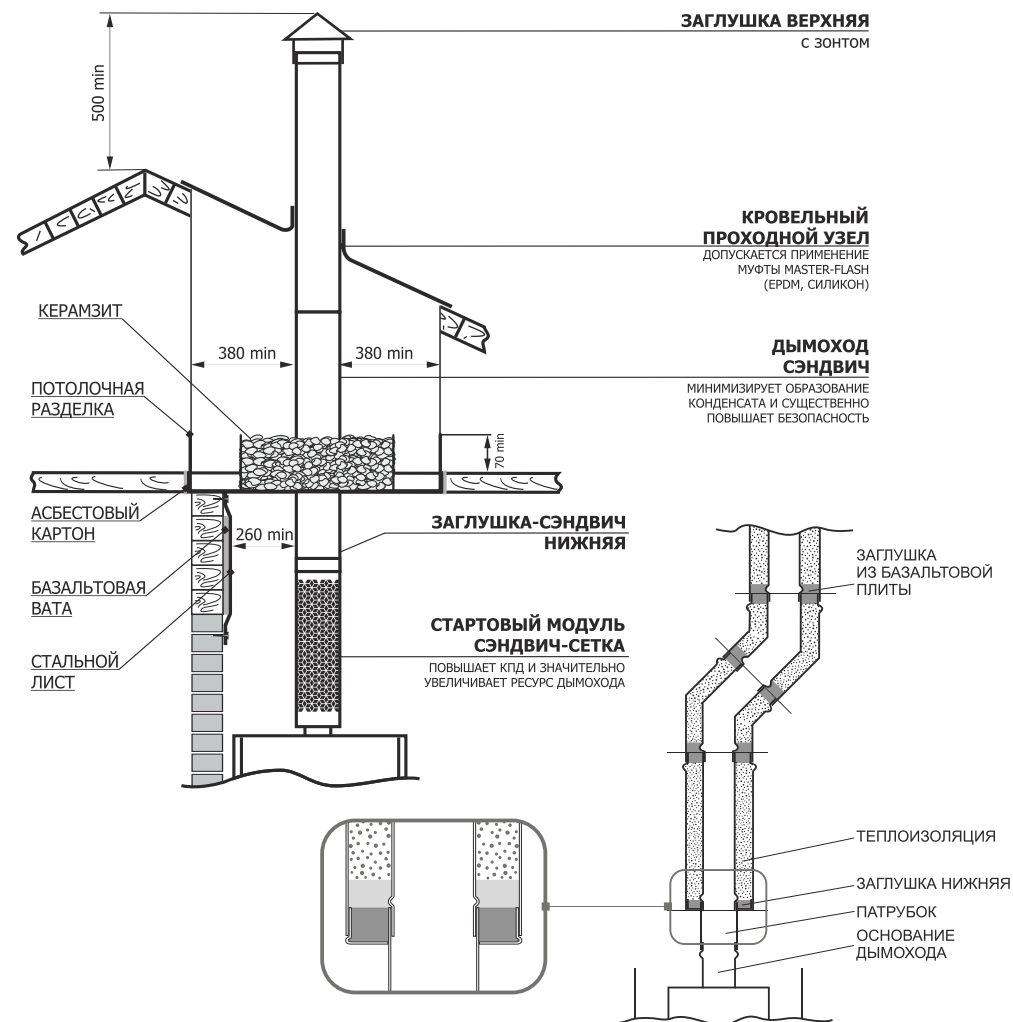
Схема установки «сэндвича» с применением отводов
